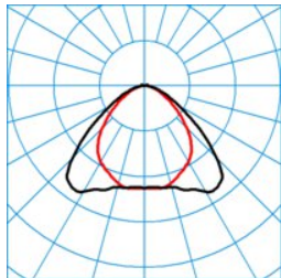
ELINE HE LVW120 827 L225 2 50 ■ C0 - C180 DIN 5040 = A40 UGR 1 = 24,4 UGR q = 25,2 UTE = 0,98 D + 0,02 T 0,90 1,50 CEN Flux Code = 53 86 97 98 100 0 0 33 2
