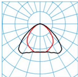
ELINE HE LVW120 865 L225 3 50 ■ C0 - C180 DIN 5040 2 = A40 UGR 1 2 = 24,6 UGR q 2 = 25,4 UTE 2 = 0,98 D + 0,02 T 0,90 1,50 CEN Flux Code 2 = 53 86 97 98 100 0 0 33 2
