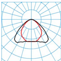
ELINE HE LVW120 840 L225 4 50 ■ C0 - C180 DIN 5040 3 = A40 UGR 1 3 = 24,4 UGR q 3 = 25,2 UTE 3 = 0,98 D + 0,02 T 0,90 1,50 CEN Flux Code 3 = 53 86 97 98 100 0 0 33 2
