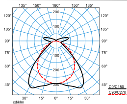
Tugra 15 PW 50-840 ET EB3 23 TX777110
