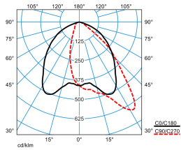
Jovie 70-AM3L-12-150-730-CLO-B
