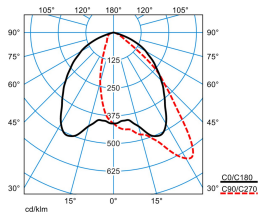
Jovie 70-AM3L-12-150-730-CLO-E
