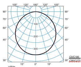
Olisq QWD3 DW 30-840 ETBLE +DMR IP54 + Olisq QWD3 ZDR 1/1 01 TX461709
