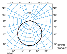
Olisq QWD3 DW 30-840 ETBLE +DMR IP54 + Olisq QWD3 ZDR 1/2 01 TX461763
