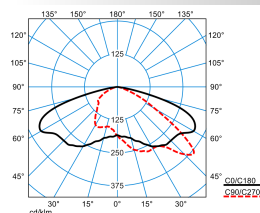
LnPlus 40-AB7L-SLR1/10000-722 8G1 ET (CLO initial value)
