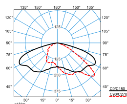
LnPlus 40-AB7L-SLR1/10000-722 8G1 ET (CLO end value)
