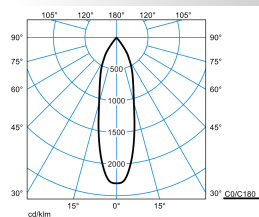
TokoP RF-MF 50-830 M41 ET 05
