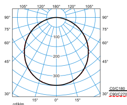
Olisq QWD2 DW 35-830 ET EB3 IK + Olisq QWD2 ZDR 1/1 01
