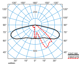
Publisca P1-AB2L/1000-730 2G1S TX047466 DIN 5040: A30 UTE: 1,00 G DLOR: 100 % ULOR: 0 % CEN Flux Code: 34 70 96 100 100
