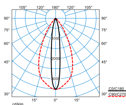
Altigo G2 C 120 SE6L/1650-830 1G1P + G2 VE IP66 24V DC 80W
