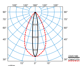
Altigo G2 C 120 SE6L/1650-830 1G1P + G2 VE IP66 24V DC 240W
