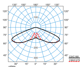
Publisca P1-RB6L/1000-730 2G1S
