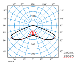
Publisca P1-RB6L/1000-730 2G1S ETDD (CLO end value)
