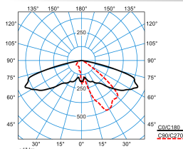
Publisca P1W-AB2L-LR/3200-740 4G1S ET (CLO initial value)
