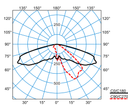
Publisca P1W-AB2L-LR/3200-740 4G1S ET (CLO end value)
