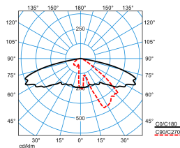
Publisca P1W-AB2L-LRA/1200-740 2G1S ET (CLO end value)
