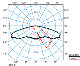
Publisca P1W-AB2L-LRA/1200-740 2G1S ET (CLO initial value)
