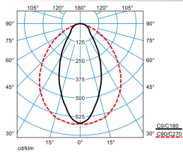
Nextrema G3 TB 8000-840 ETDD +LV TX770453
