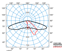
Publisca P1W-AB2L-LR/2200-730 3G1S ET (CLO end value)
