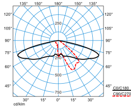
Publisca P1W-AB2L-LR/2200-730 3G1S ET (CLO initial value)
