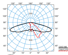
Publisca P1W-AB2L-LR/2200-730 3G1S ET (CLO end value)
