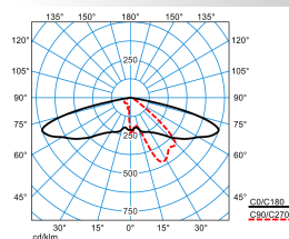
Publisca P1W-AB2L-LR/2200-730 3G1S ET (CLO initial value)
