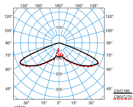
Publisca P1W-RB6L-LRA/2200-740 3G1S ET (CLO end value)
