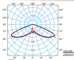
Publisca P1W-RB6L-LRA/2200-740 3G1S ET (CLO initial value)
