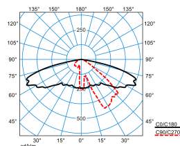
Publisca P1W-AB2L-LRA/1500-730 2G1S ET (CLO end value)
