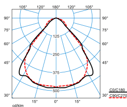
SFlow D3-L MRW LED4000-8TW ETDD8 LLWM 03 (DSU)
