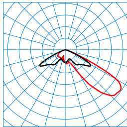
LnPlus 70-AM19L/62000-740 48G1 ETDD (CLO end value) TX376992 ■ C0 - C180 ■ C90 - C270 DIN 5040: A30 UTE: 1,00 J DLOR: 100 % ULOR: 0 % CEN Flux Code: 26 78 99 100 100
