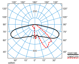
Publisca P2-AB2L-LRA/2000-730 3G1S ET (CLO initial value)
