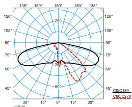
Publisca P2-AB2L-LRA/2000-730 3G1S ET (CLO end value)
