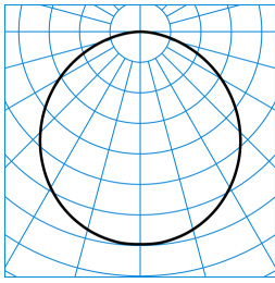
Olisq RWD2 DW 40-830 ET PC + Olisq RWD2 ZDR 1/1 01 TX425950
