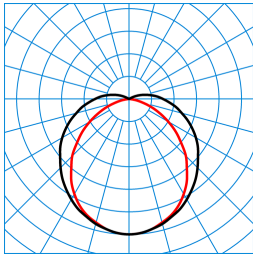
Kratex HE 1200 40-840 ET PC EB3 TX774577
