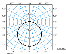
Olisq RWD2 DW 40-830 ET EB3 PC + Olisq RWD2 ZDR 1/2 05 TX428720
