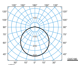
Olisq RWD2 DW 40-830 ET EB3 PC + Olisq RWD2 C 01 TX425807
