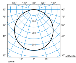
Olisq RWD2 DW 40-830 ET EB3 PC + Olisq RWD2 ZDR 1/1 01
