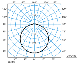
Olisq RWD2 DW 40-830 ET EB3 PC + Olisq RWD2 ZDR 1/2 01 TX426079
