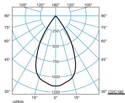
E-Line PRO 78 BV G2 RF-VFL 20-830 M33 ET 01 01
