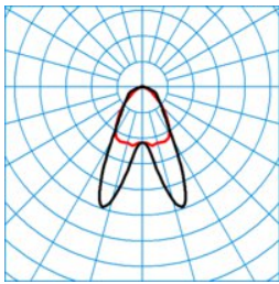
ELINE FL LDAN140 830 L225 1 20
