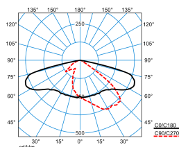
LnPlus 40-AB7L/18000-740 12G1 ETDD (CLO initial value) TX377555
