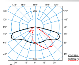
LnPlus 40-AB7L/18000-740 12G1 ETDD (CLO end value) TX377490
