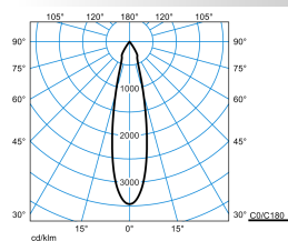
QuiraP G2 RF-MF 40-BC M51 ETDD 01
