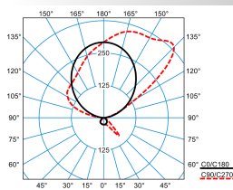
Luceos S G3 PAW-IA 170-9TW ETDS KL 03 (DWW)
