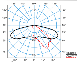
Cuvia 60-AB2L/6800-740 8G1S ET
