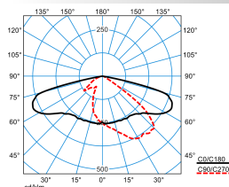
LnPlus 40-AB7L-SLR1/2200-727 2G1 ET (CLO end value) TX377368
