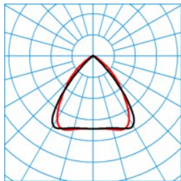
ELINE FL LN180 830 L225 1 20
