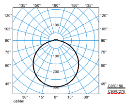
Olisq QWD2 DW 20-8TW ETDD8 IP54 + QWD2 ZDR 1/2 01 (DWW) TX873149
