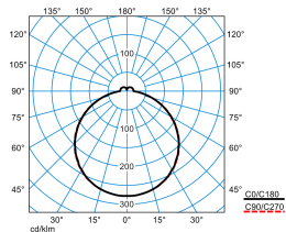
Olisq QWD2 DW 20-8TW ETDD8 IP54 (DSU) TX873136
