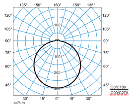
Olisq QWD2 DW 20-8TW ETDD8 IP54 + QWD2 ZDR 1/2 03 (DWW) TX873152
