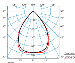
LPCV 3P2-ST L-W 05 45-8TW S96 ETBLE 01 (DSU)
