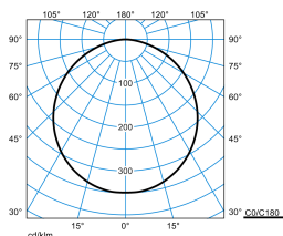
Olisq RWD4 DW 40-8TW ETDD8 + Olisq RWD4 ZDR 1/1 03 (DSU)
