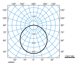
Olisq RWD4 DW 40-8TW ETDD8 + Olisq RWD4 C 01 (DCW)
