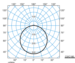
Olisq RWD4 DW 40-8TW ETDD8 + Olisq RWD4 ZDR 1/2 01 (DCW)
