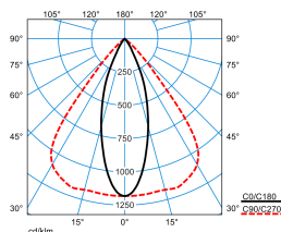
YVTW 3P L-OVL 30-EW M48 ET 05 (LEO1)
