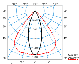
YVTW 3P L-OVL 30-EW M48 ET 05 (LEO2)
