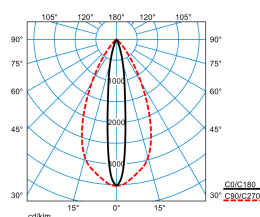
Altigo G2 10 SE6L/300-830 1G1P + VE IP66 24V DC 60W
