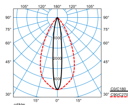
Altigo G2 10 SE6L/300-830 1G1P + G2 VE IP66 24V DC 240W
