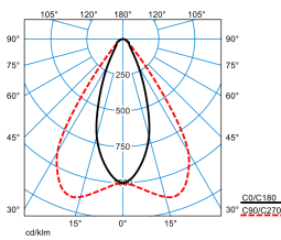
E-Line PRO 78IP50 MironaF HR 270-840 ET L225 01 ESG Blank (LEO2)
