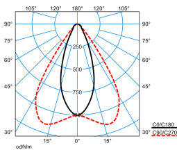
E-Line PRO 78IP50 MironaF HR 270-840 ET L225 01 ESG 01 (LEO2)
