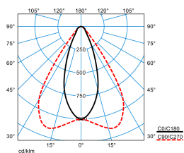
E-Line PRO 78IP50 MironaF HR 270-840 ET L225 01 ESG Blank (LEO3)
