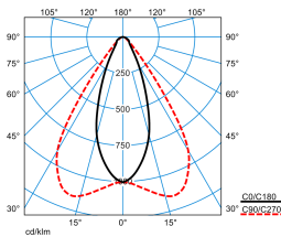
E-Line PRO 78IP50 MironaF HR 270-840 ET L150 01 ESG 01 IP50 (LEO1)
