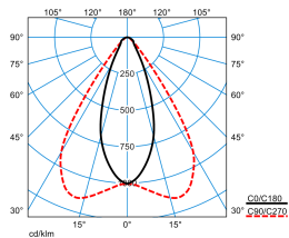
E-Line PRO 78IP50 MironaF HR 270-840 ET L225 01 ESG Blank (LEO1)
