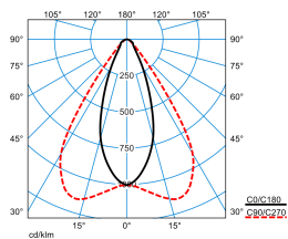
E-Line PRO 78IP50 MironaF HR 270-840 ET L150 01 ESG 01 IP50 (LEO2)
