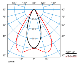
E-Line PRO 78IP50 MironaF HR 270-840 ET L150 01 ESG Blank IP50 (LEO1)
