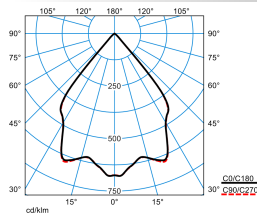
LPCV 3P2 L-W19 01 80-840 K04 ET 01
