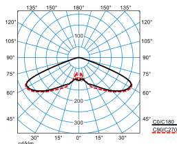
Publisca P2-RB6L-LR/4600-730 6G1S ET (CLO initial value)
