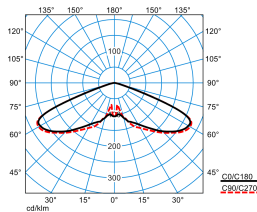
Publisca P2-RB6L-LR/4600-730 6G1S
