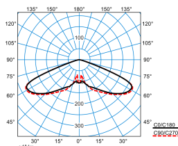
Publisca P2-RB6L-LR/4600-730 6G1S ET (CLO end value)
