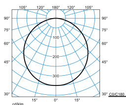
Olisq RWD4 DW 40-8TW ETBLE +CAS-S IP54 + Olisq RWD4 ZDR 1/1 05 (DSU)
