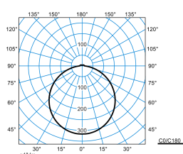
Olisq RWD4 DW 40-8TW ETBLE +CAS-S IP54 + Olisq RWD4 ZDR 1/2 05 (DCW)
