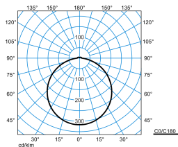
Olisq RWD4 DW 40-8TW ETBLE +CAS-S IP54 + Olisq RWD4 ZDR 1/2 03 (DSU)
