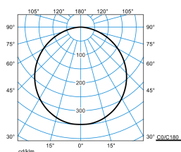
Olisq RWD4 DW 40-8TW ETBLE +CAS-S IP54 + Olisq RWD4 ZDR 1/1 05 (DCW)
