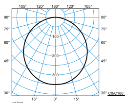
Olisq RWD4 DW 40-8TW ETBLE +CAS-S IP54 + Olisq RWD4 ZDR 1/1 01 (DWW)
