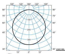
Olisq RWD4 DW 40-8TW ETBLE +CAS-S IP54 + Olisq RWD4 ZDR 1/1 01 (DCW)
