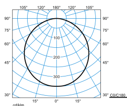
Olisq RWD4 DW 40-8TW ETBLE +CAS-S IP54 + Olisq RWD4 ZDR 1/1 03 (DWW)
