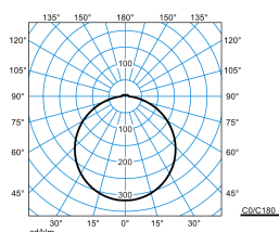
Olisq RWD4 DW 40-8TW ETBLE +CAS-S IP54 + Olisq RWD4 ZDR 1/2 03 (DCW)
