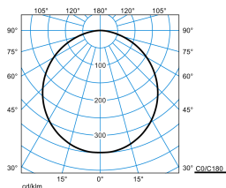
Olisq RWD4 DW 40-8TW ETBLE +CAS-S IP54 + Olisq RWD4 ZDR 1/1 05 (DWW)
