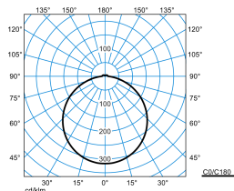
Olisq RWD4 DW 40-8TW ETBLE +CAS-S IP54 + Olisq RWD4 ZDR 1/2 05 (DWW)
