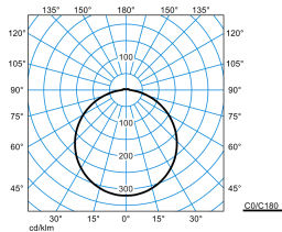
Olisq RWD4 DW 40-8TW ETBLE +CAS-S IP54 + Olisq RWD4 C 01 (DSU)
