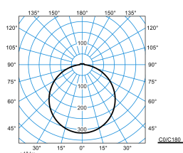
Olisq RWD4 DW 40-8TW ETBLE +CAS-S IP54 + Olisq RWD4 ZDR 1/2 01 (DCW)
