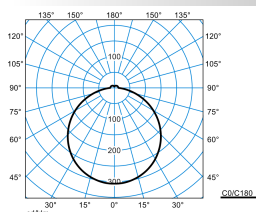
Olisq RWD4 DW 40-8TW ETBLE +CAS-S IP54 (DWW)
