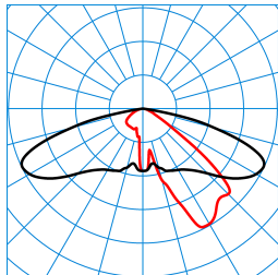
Publisca P1-AB2L-LRA/4600-740 6G1S ET (CLO end value) TX301834 ■ C0 - C180 ■ C90 - C270 DIN 5040: A30 UTE: 1,00 G DLOR: 100 % ULOR: 0 % CEN Flux Code: 35 74 97 100 100
