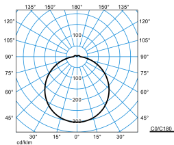
Olisq RWD2 DW 20-8TW ETDD8 IP54 + RWD2 ZDR 1/2 03 (DSU)
