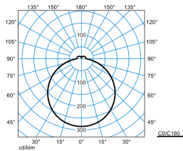
Olisq RWD2 DW 20-8TW ETDD8 IP54 (DSU)
