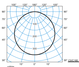
Olisq RWD2 DW 20-8TW ETDD8 IP54 + RWD2 ZVF 03 (DSU)
