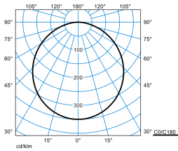
Olisq RWD2 DW 20-8TW ETDD8 IP54 + RWD2 ZVF 01 (DSU)
