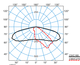
LIQ 50N-AB2L-LR/1500-730 2G1 ET (CLO end value)
