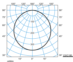
Olisq RWD3 DW 50-840 ETDD IP54 + Olisq RWD3 ZVF 03
