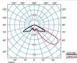
LnPlus 70-AM19L-SLR1/51000-740 48G1 ET (CLO initial value)
