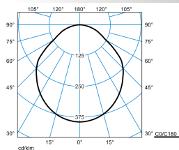
Onplana D09 OTA25 3000-830 ET 01 TX771892
