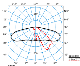
Publisca P2-AB2L-LR/1000-730 2G1S ET (CLO end value) TX301282 DIN 5040: A30 UTE: 1,00 G DLOR: 100 % ULOR: 0 % CEN Flux Code: 34 70 96 100 100
