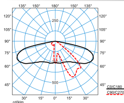
Publisca P2-AB2L-LR/1000-730 2G1S TX047731 DIN 5040: A30 UTE: 1,00 G DLOR: 100 % ULOR: 0 % CEN Flux Code: 34 70 96 100 100
