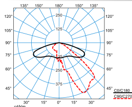
Publisca P2-AB2L/3500-730 4G1S TX047720 DIN 5040: A30 UTE: 1,00 G DLOR: 100 % ULOR: 0 % CEN Flux Code: 35 73 97 100 100
