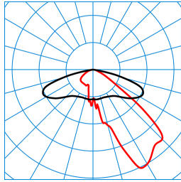
Publisca P2-AB2L/3500-730 4G1S TX047720 ■ C0 - C180 ■ C90 - C270 DIN 5040: A30 UTE: 1,00 G DLOR: 100 % ULOR: 0 % CEN Flux Code: 35 73 97 100 100
