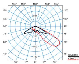
LnPlus 70-AM19L-SLR2/51000-740 48G1 ET (CLO end value)
