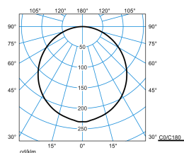
Varisto600 6000-830 S07 ET 01 (LEO7)
