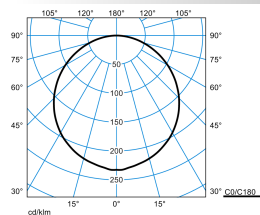
Varisto600 6000-830 S07 ET 01 (LEO12)
