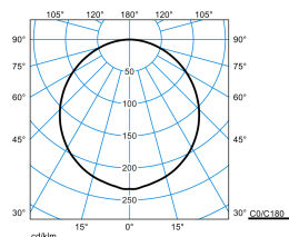
Varisto600 6000-830 S07 ET 01 (LEO5)
