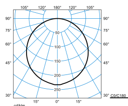
Varisto600 6000-830 S07 ET 01 (LEO9)
