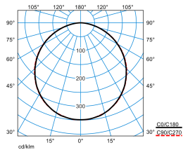
Olisq QWD3 DW 45-840 ETBLE +DMM IP54 IK + Olisq QWD3 ZDR 1/1 05
