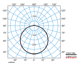
Olisq QWD3 DW 45-840 ETBLE +DMM IP54 IK + Olisq QWD3 ZDR 1/2 03
