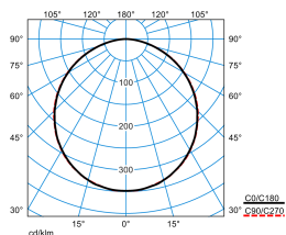
Olisq QWD3 DW 45-840 ETBLE +DMM IP54 IK + Olisq QWD3 ZDR 1/1 01
